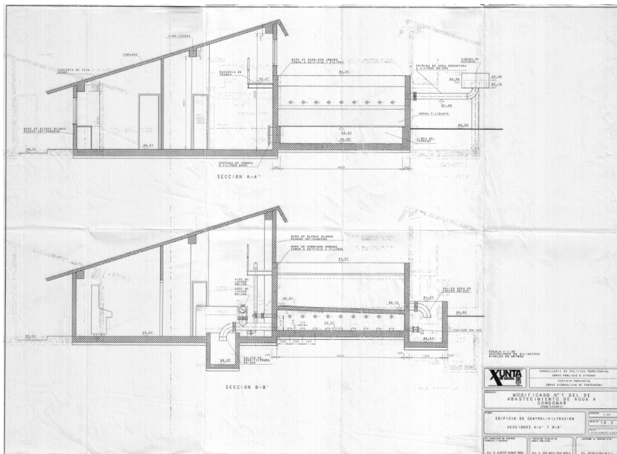
Esquema 6: Plano secciones A-A y B-B edificio y filtros ETAP
