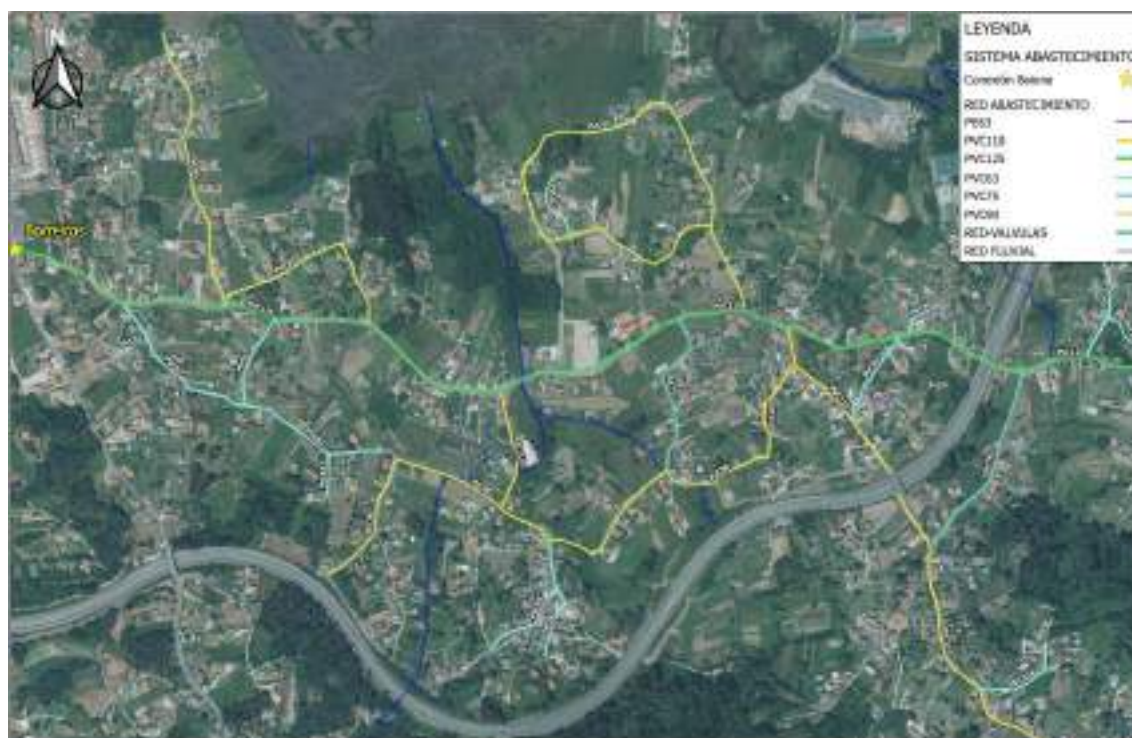
Figura 32: Conexión con red abastecimiento municipal de Baiona en zona Borreiros
