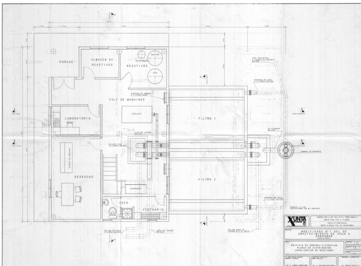
Esquema 5: Plano proyecto edificio y filtros ETAP
