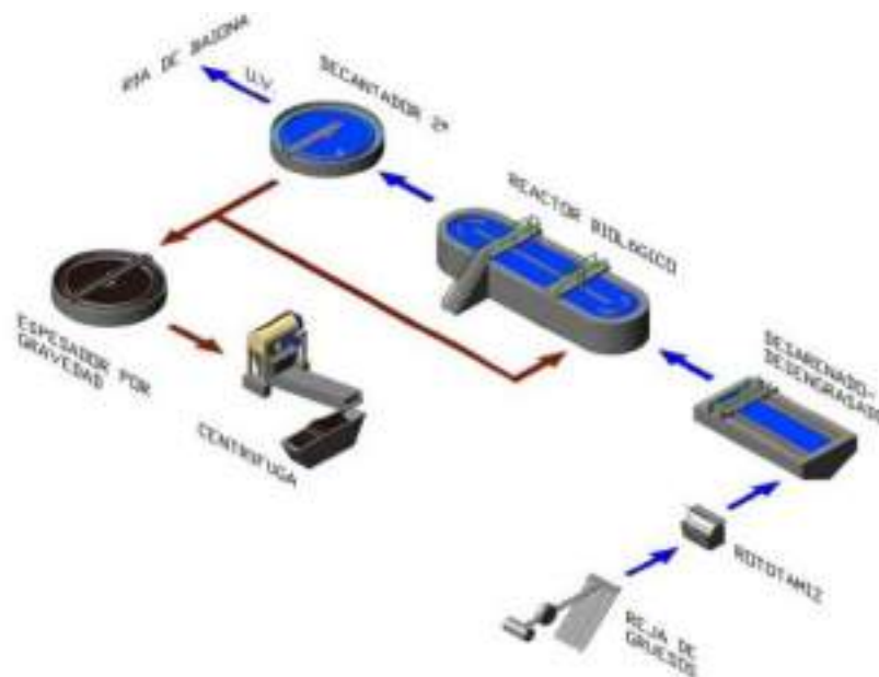
Figura 37. Esquema proceso de depuración EDAR Gondomar.
