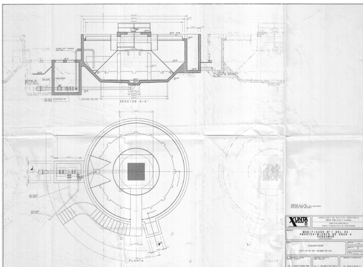
Foto 12: Plano de proyecto decantador en ETAP
