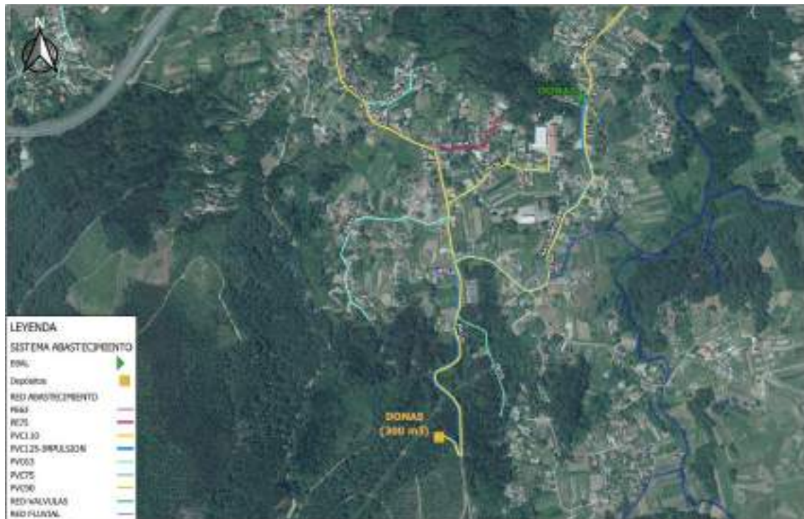
Figura 26: EBAL de Donas
