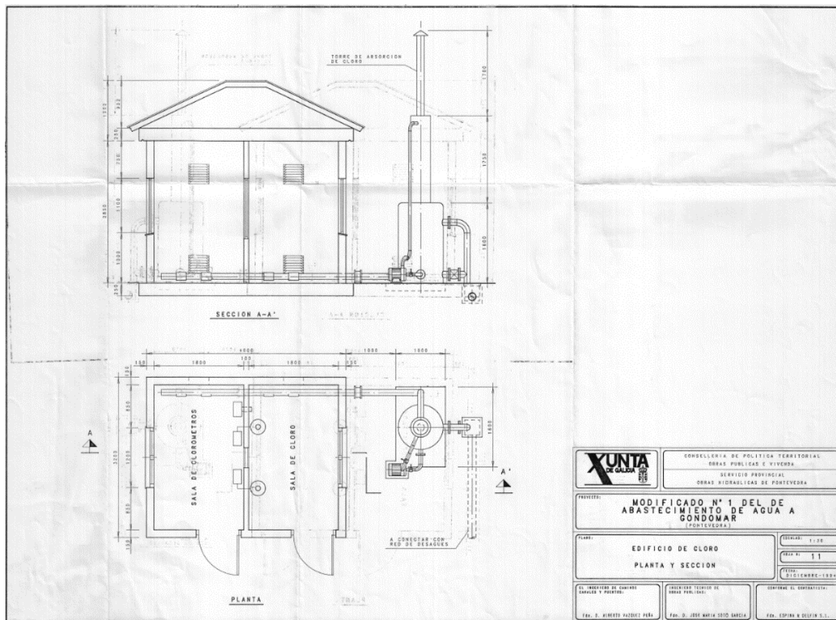
Esquema 8: Plano proyecto caseta cloro en ETAP
