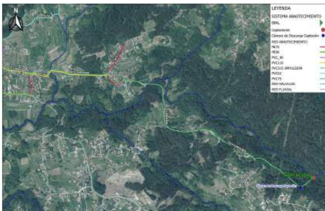
Figura 14: Captación de Gondomar no río Touteiras/Miñor
