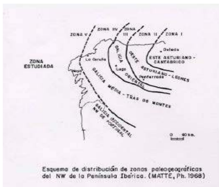
Figura 8. División del Macizo Ibérico según Matte (1968).
