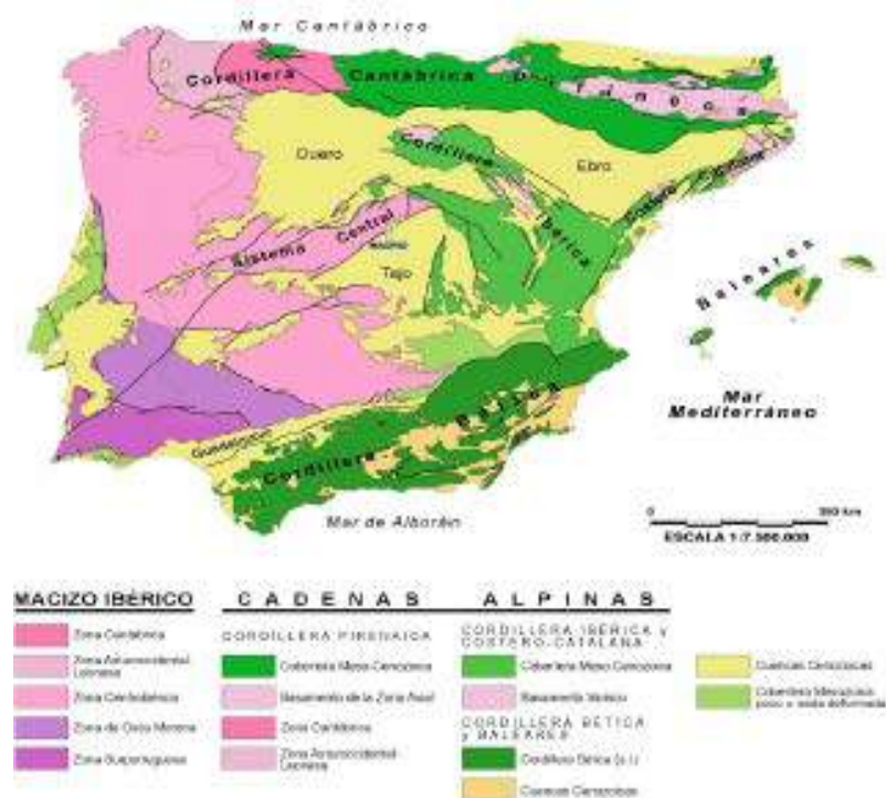
Figura 7. Compartimentación estructural de la Península Ibérica.
