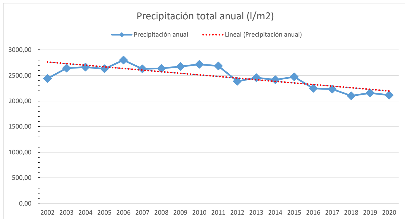
Figura 6. Precipitación total anual en la estación del Monte Aloia (Tui).
