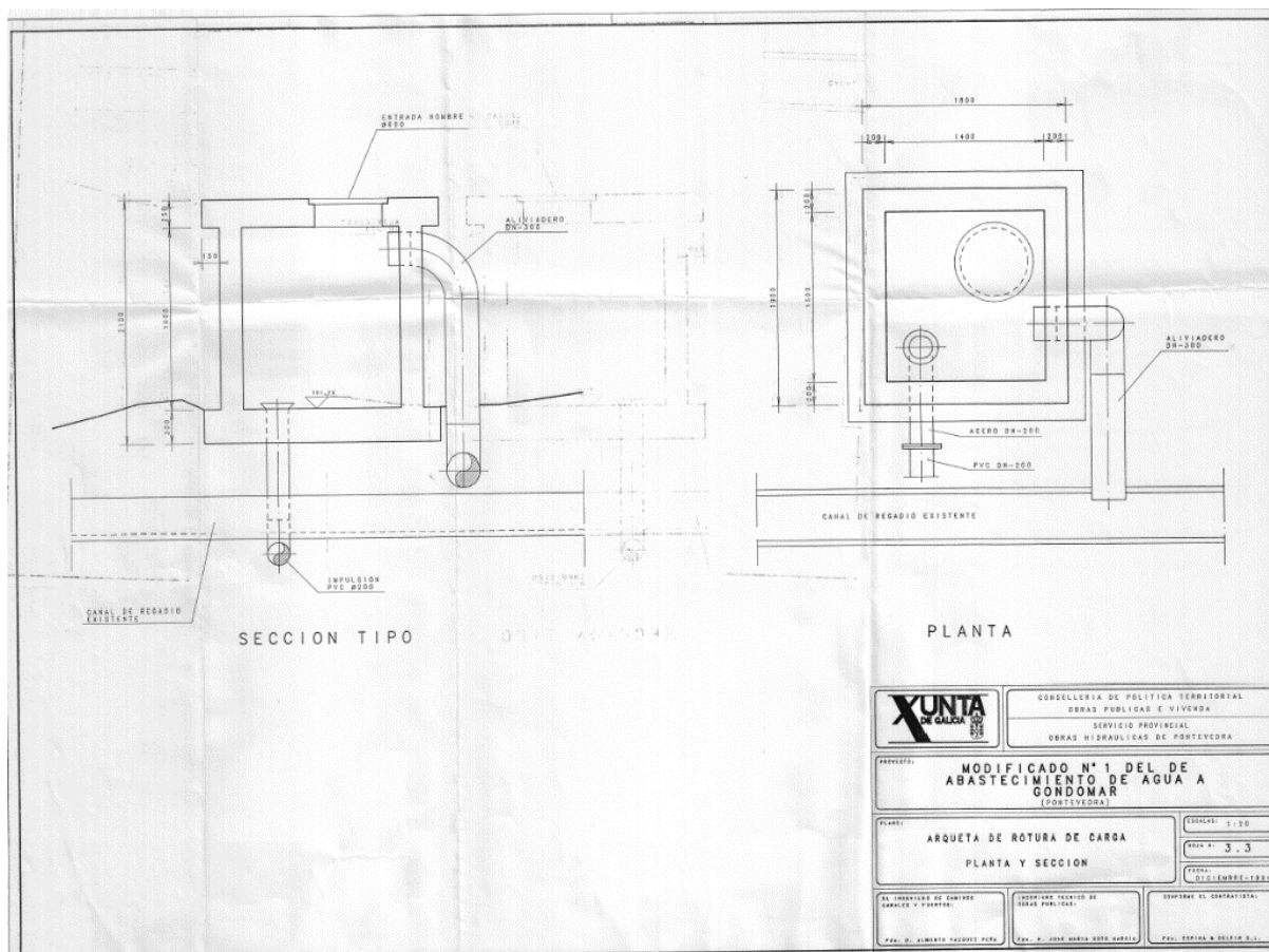
Esquema 3: Plano de proyecto de cámara de descarga impulsión captación de Gondomar
