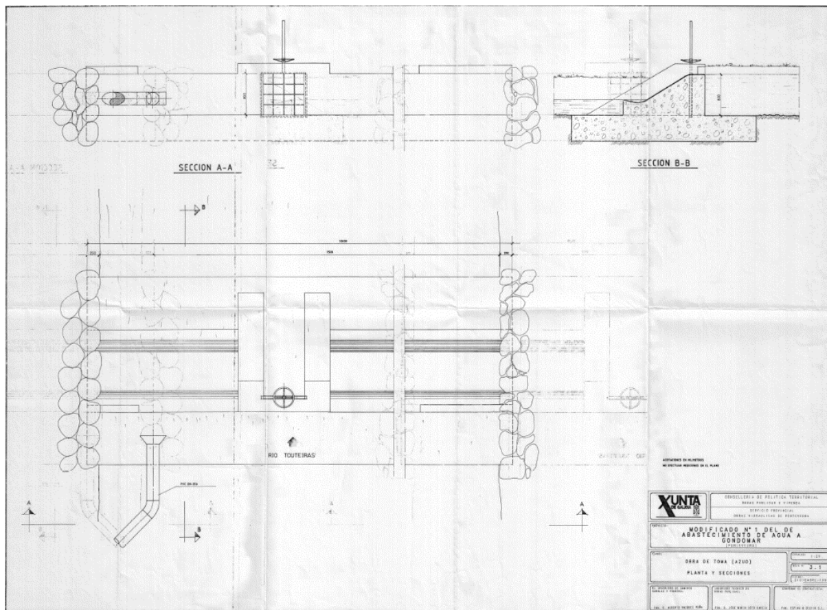
Esquema 1: Plano de proyecto de azud de captación
