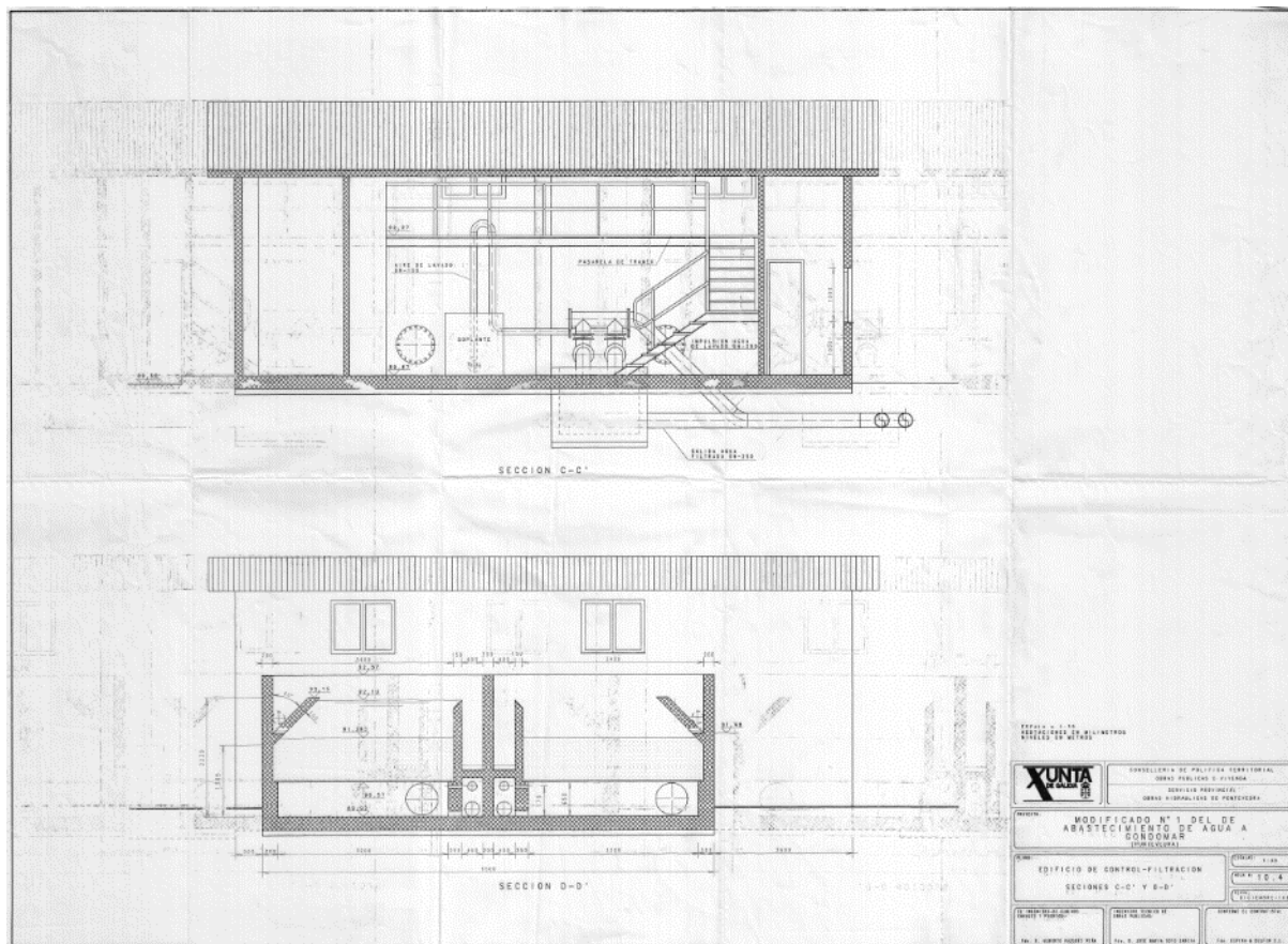
Esquema 7: Plano secciones C-C y D-D edificio y filtros ETAP
