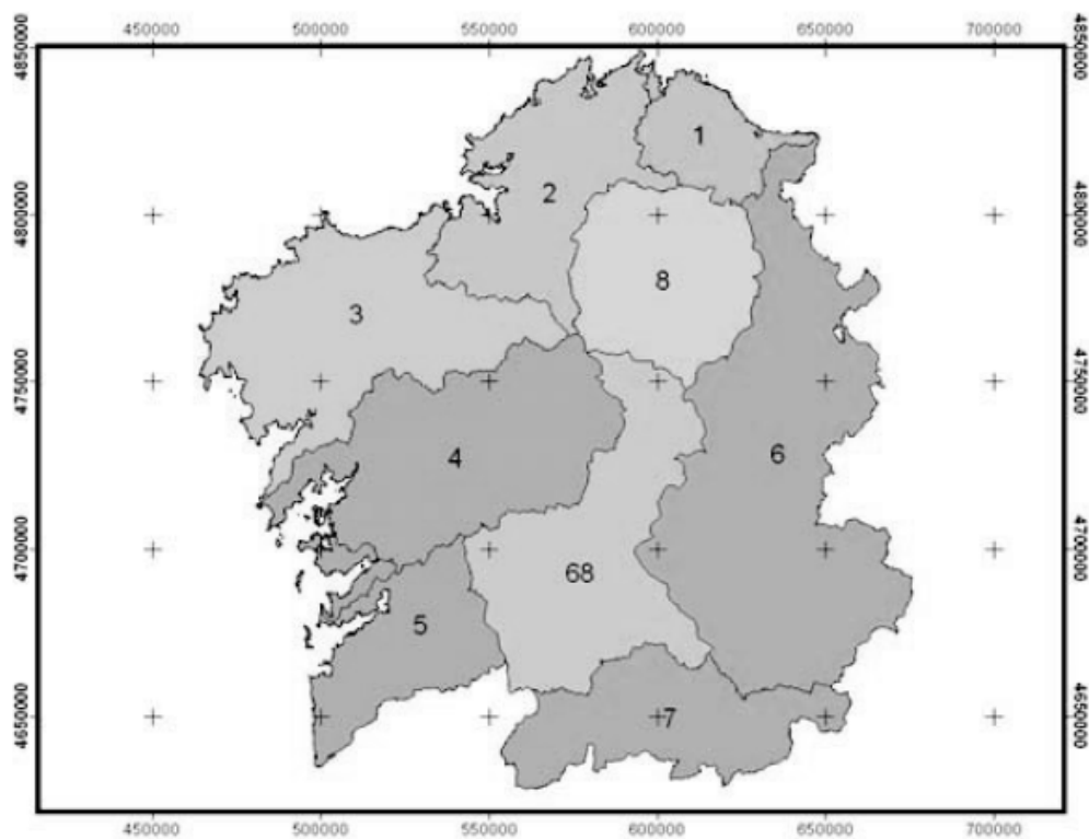
Figura 44. Zonas para la obtención del coeficiente de estiaje.
