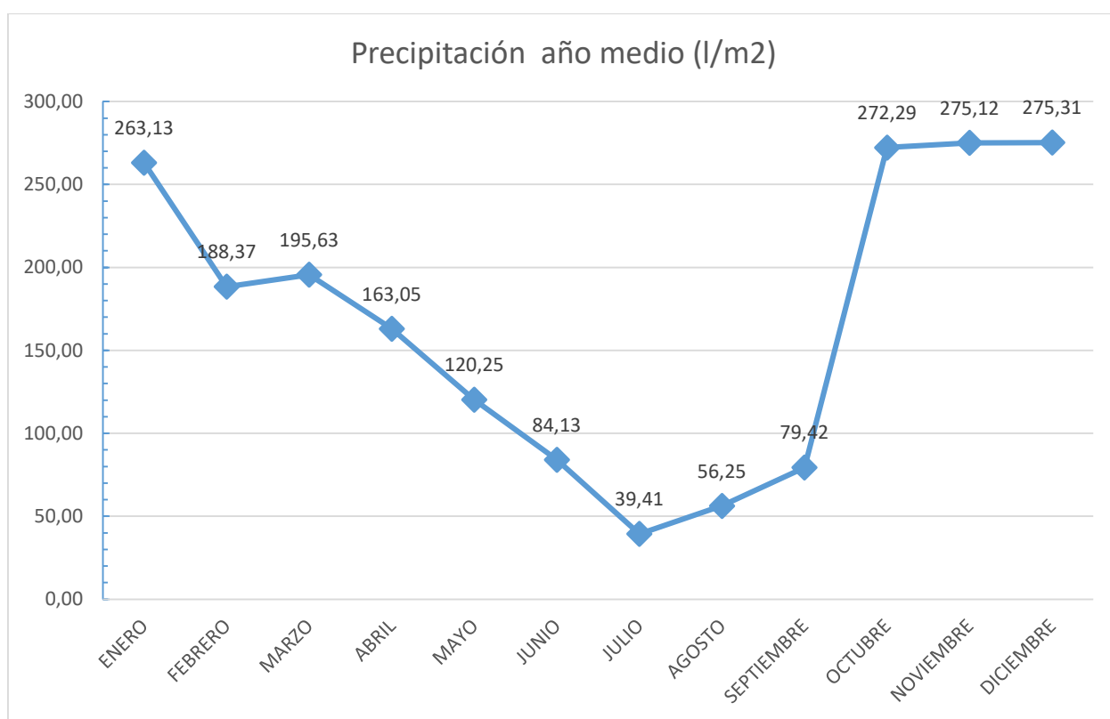
Figura 5. Precipitación media mensual en la estación del Monte Aloia (Tui).
