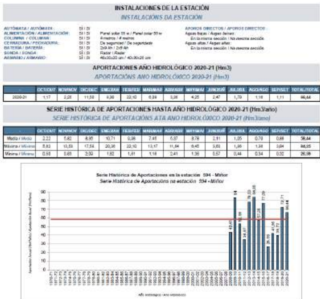
Figura 43. Series históricas de caudales.
