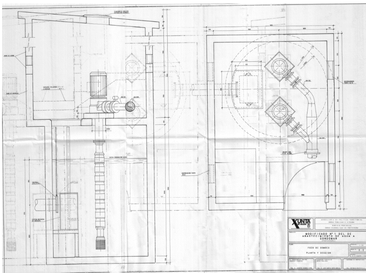
Esquema 2: Plano de proyecto de pozo de bombeo de captación de Gondomar
